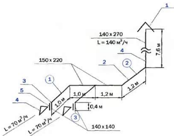
Рис. 8.7. Расчетная аксонометрическая схема к примеру: 1 — вытяжной зонт; 2 — утепленный шлакогипсовый короб; 3 — кирпичный канал; 4 — шахта кирпичная, оштукатуренная по сетке; 5 — решетка. Цифры в кружках — нумерация участков
