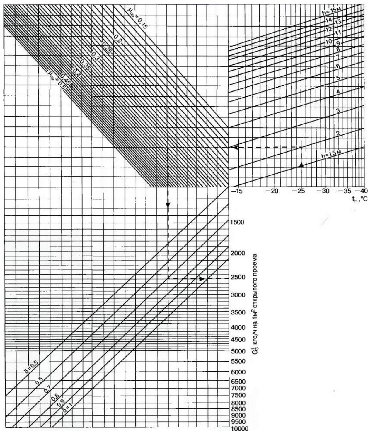
Рис. 7.3. Номограмма для определения расхода воздуха завесы шиберующего типа
