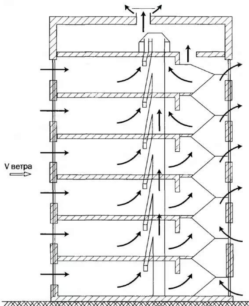
Рис. 1.1. Формирование воздушных потоков в многоэтажном здании с естественной вентиляцией
