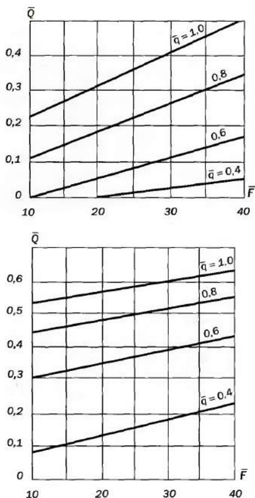
Рис. 7.4. График для определения потерь тепла с частью струи завесы шибрующего типа, уходящей наружу: а — для боковой завесы; б — для нижней завесы
