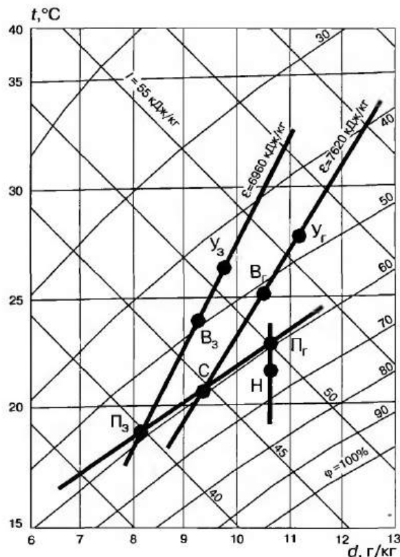
Рис. 6.2. Пример построения процессов на l - d диаграмме
