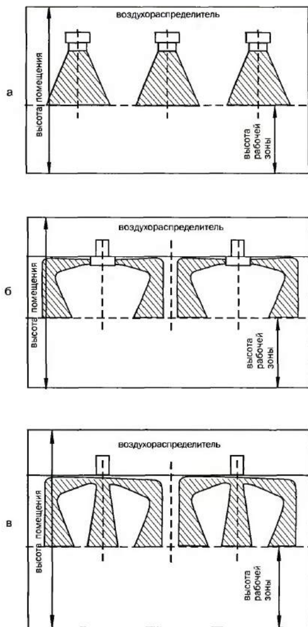
Рис. 9.4. Веерные струи:
