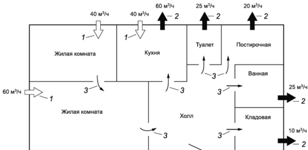
Рисунок 1 - Пример схемы организации воздухообмена в квартире
